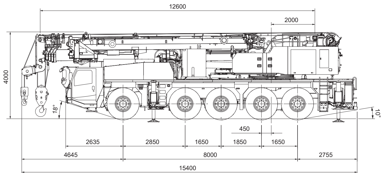
※構内走行姿勢図 (16tカウンターウェイト装着時)
